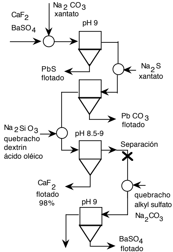
Figura 12 : Separación de fluorita y barita
